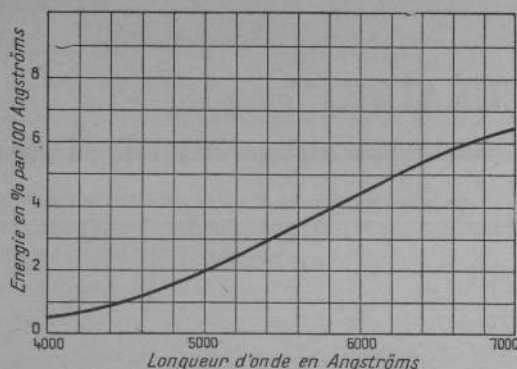
Fig. 2. — Graphique obtenu avec une lampe à incandescence.
