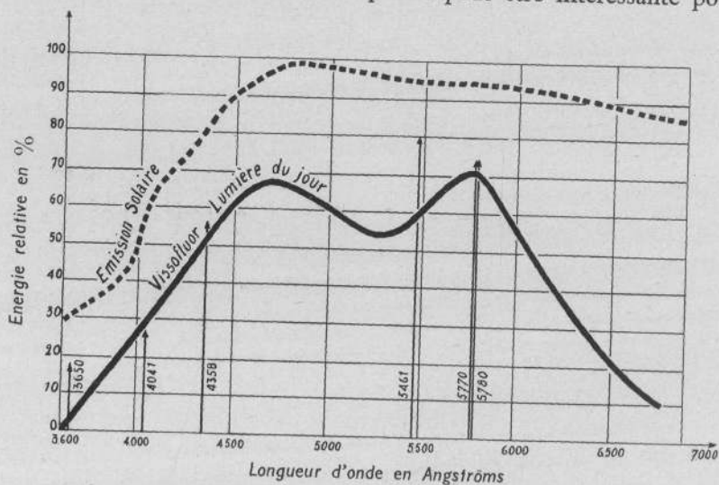
Fig. 4. — Spectre d'émission d'un tube « lumière du jour » Visseaux.
