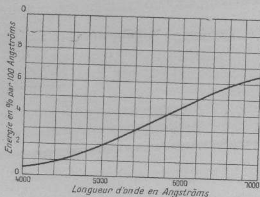
Fig. 2. — Graphique obtenu avec une lampe à incandescence.
