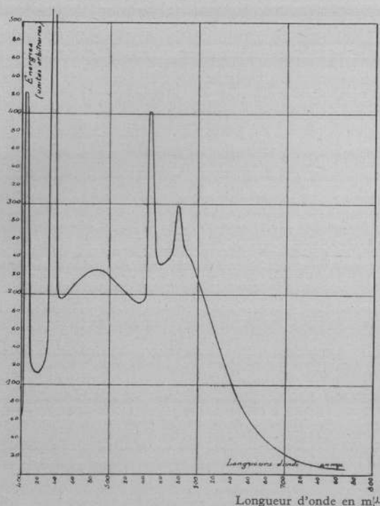
Fig. 5. — Spectre d'émission d'un tube « lumière du jour » Sylvania.
