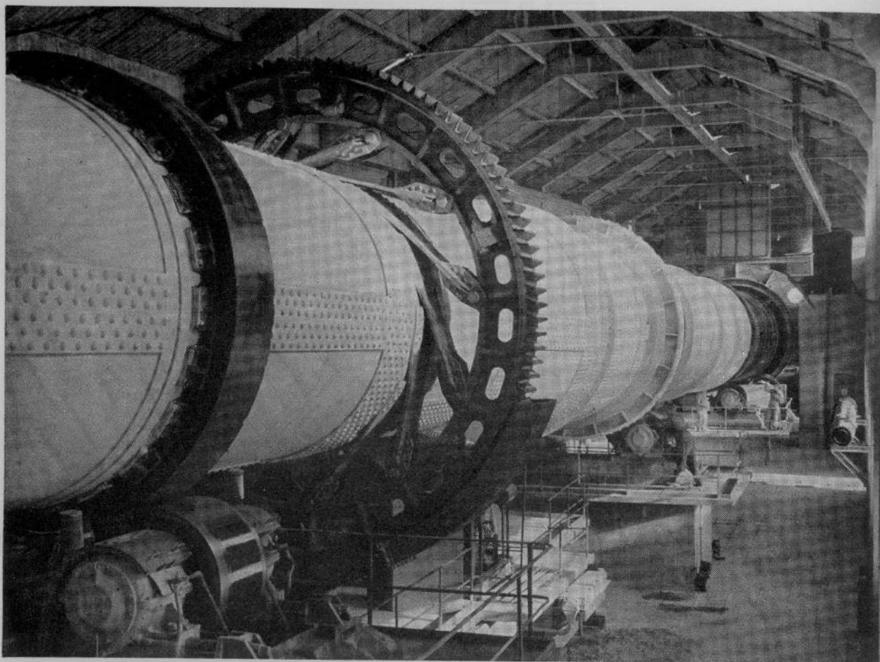
Il più grande forno da cemento del mondo lavora giorno e notte nelle fabbriche di Aalborg.
