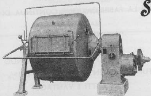
Zangola in acciaio inossidabile che impasta il burro nel vuoto.
