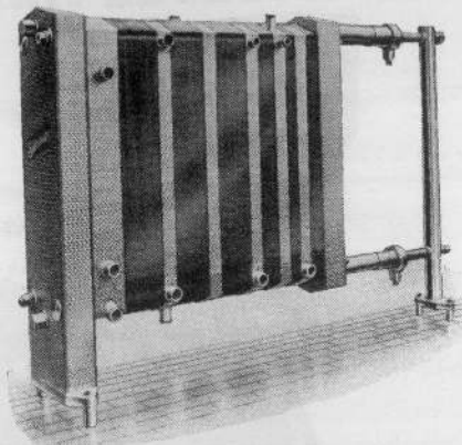
Apparecchio a piastre di acciaio inossidabile con piastre "a multiturbulenza"
