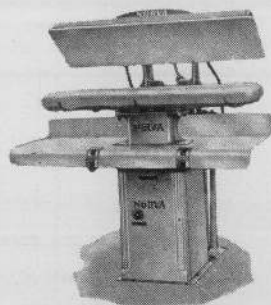
Macchina stiratrice per lavanderie
