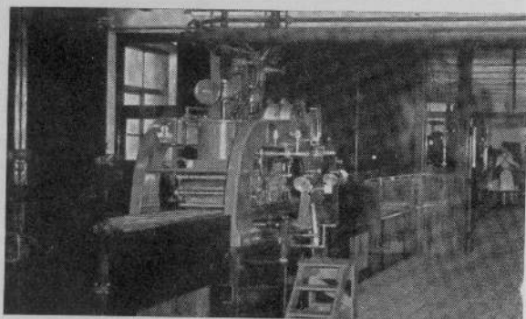
Impianto continuo automatico di modellaggio per cioccolato puro e con ripieno
