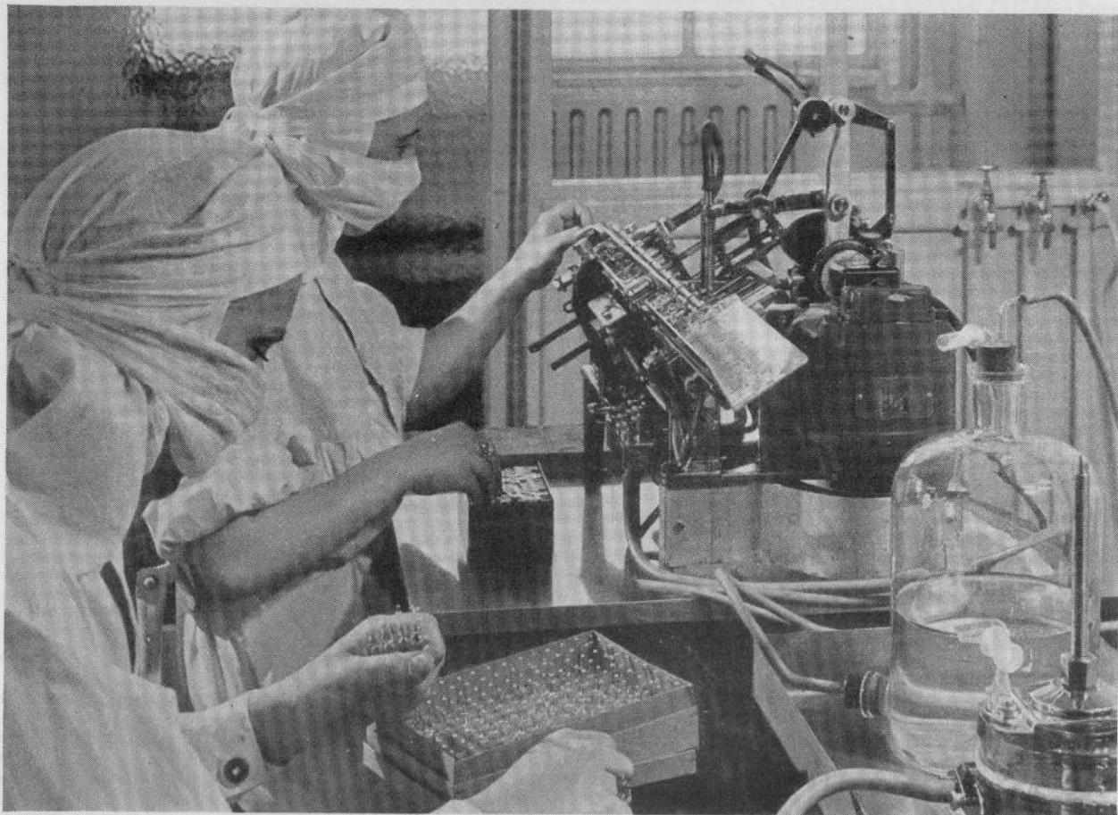
Apparecchio per il riempimento semiautomatico delle fiale. Vengono adottate tutte le precauzioni per garantire la asepsi.
