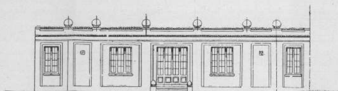
Prospetto della veranda di comunicazione tra i due Padiglioni
