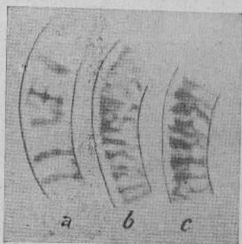
Fig. 2. — Lo stesso tratto del reticolo della figura precedente ingrandito e ripreso dalle tre osservazioni in campo oscuro ( a ), a luce ordinaria ( b ) e dopo colorazione col metodo di Feulgen.
