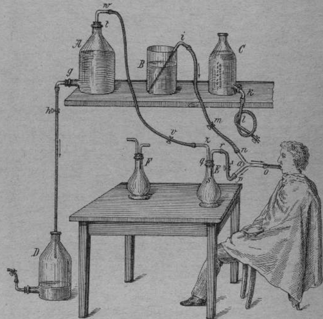
A ist eine mehrere Liter fassende Aspirationsflasche, mit gewöhnlichem Wasser vollgefüllt; am Boden derselben ist die
